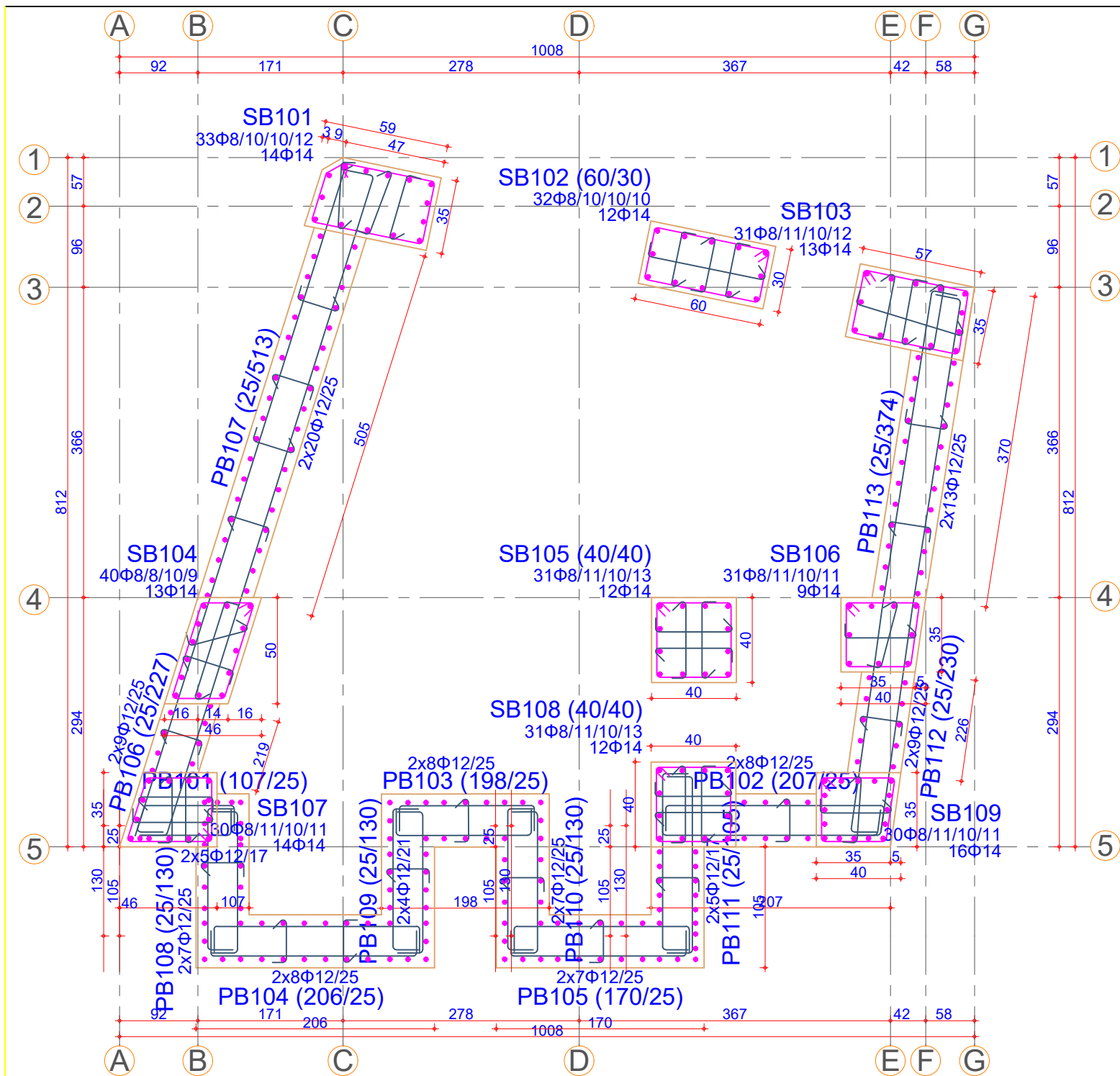
1. BODRUM Kolon Aplikasyon Planı
